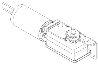
21900000 MOTOR & GEARBOX 64ZY SPROCKET UP
